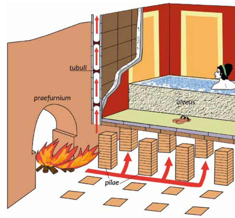
Representació d'un hipocaust a partir d'un dibuix de Jean- Pierre Adam (J. Ciurana).
